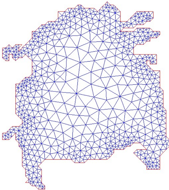
Abb. 3: Ekmangleichung
